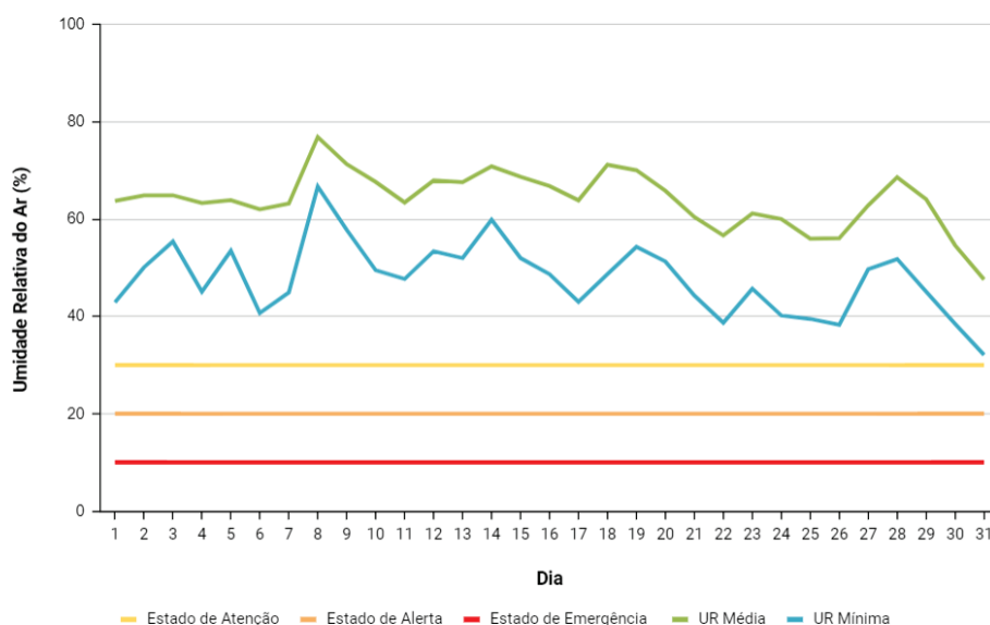
Figura 6. Umidade relativa (%) em Itabira para o mês de março
