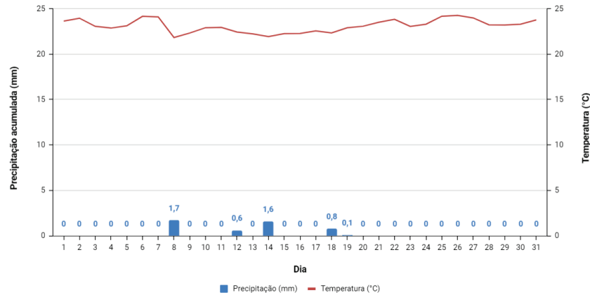
Figura 5. Precipitação diária (mm) e temperatura (°C) em Itabira para o mês de março
